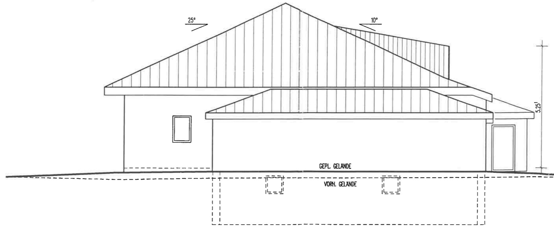
WESTANSICHT
