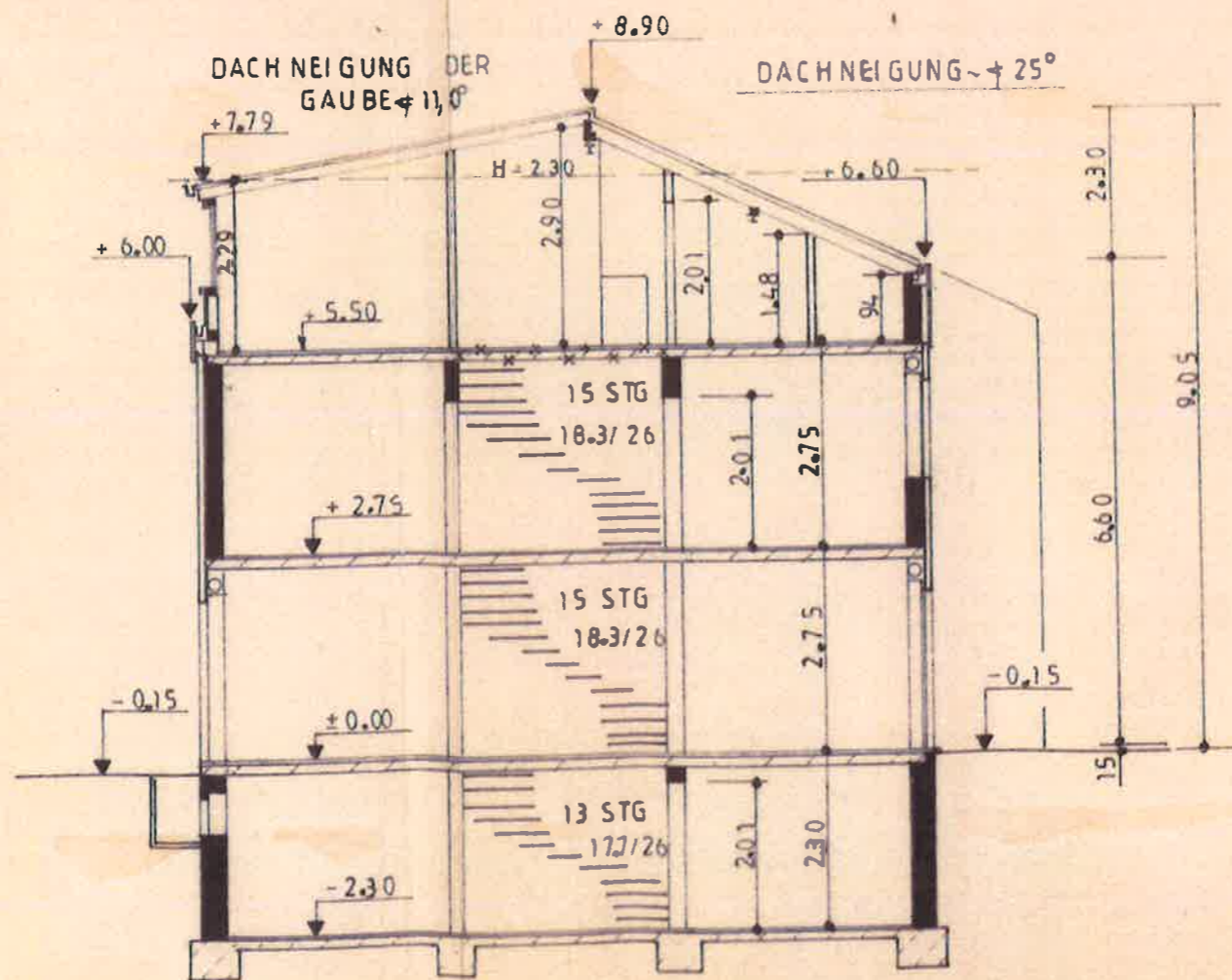
SCHNITT A-A
