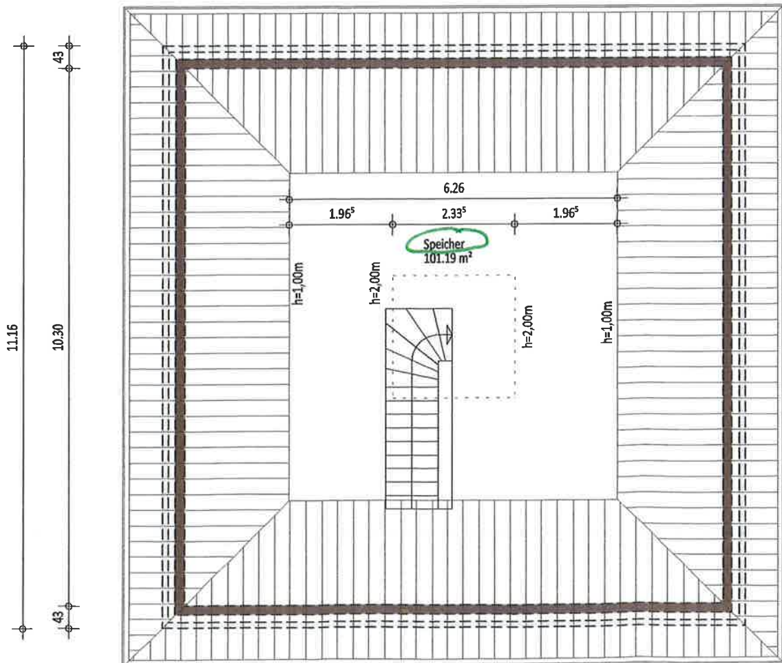
DACHGESCHOSS
