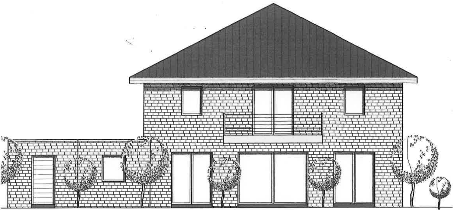
GARTENANSICHT
