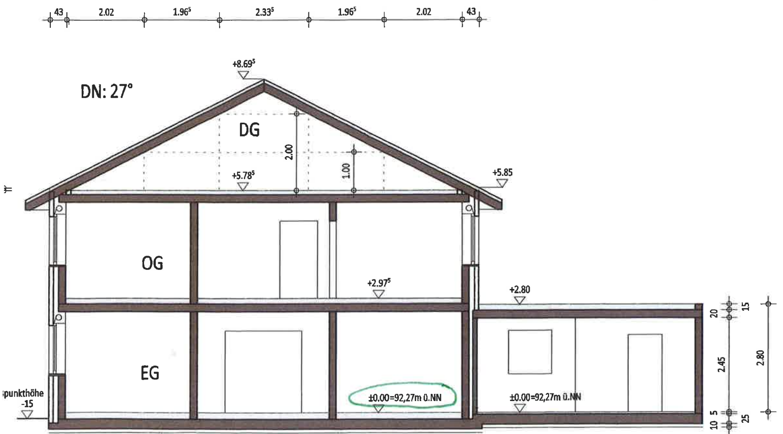
SCHNITT A-A
