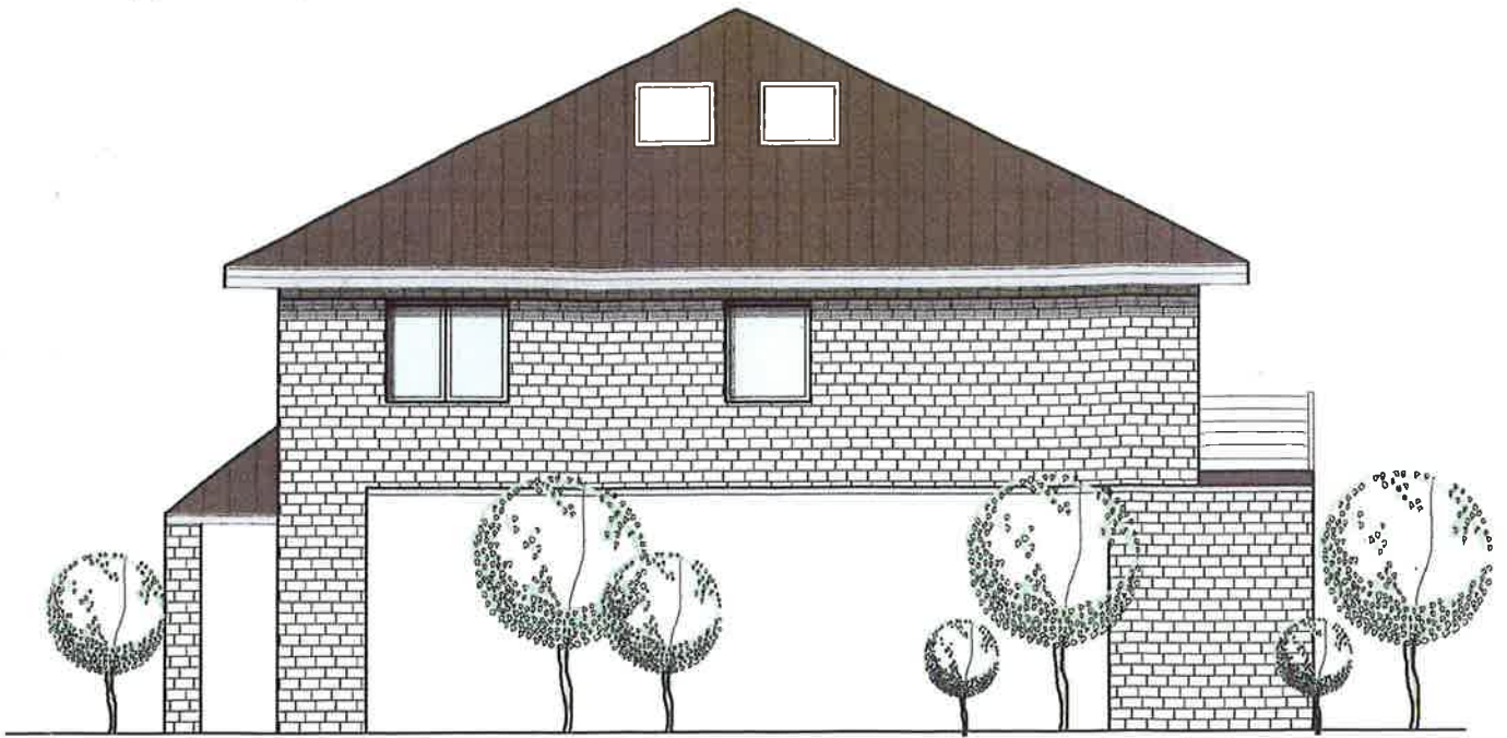
SEITENANSICHT RECHTS
